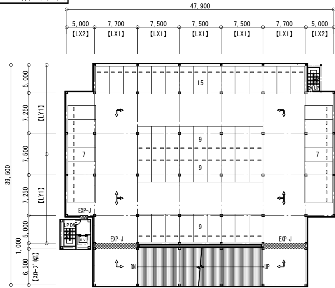
2～6階 平面図
