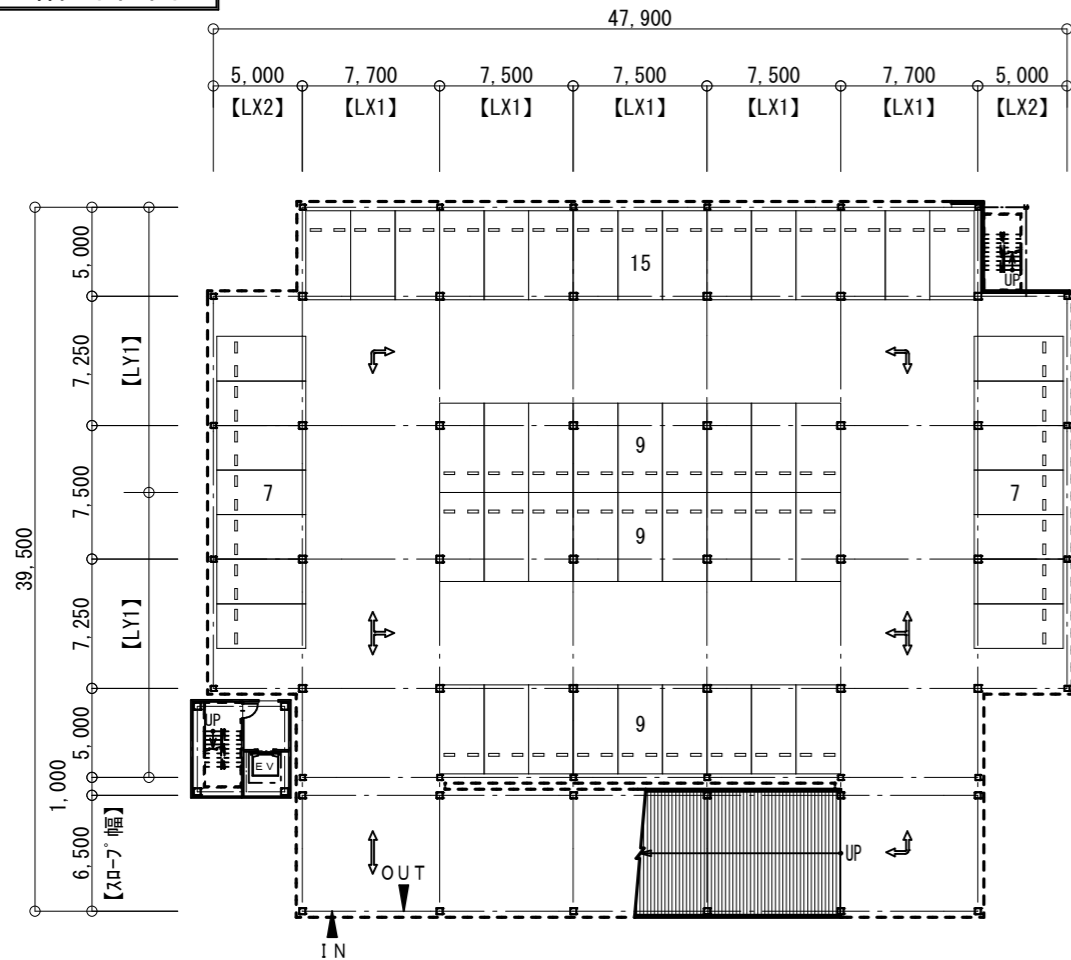
1階 平面図
